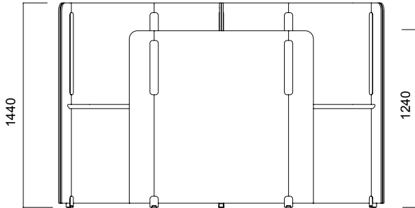
Tip 6 İgili Kademeli T Panel
