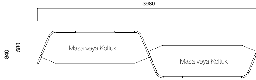
Tip 2 Açılı İkili Panel
