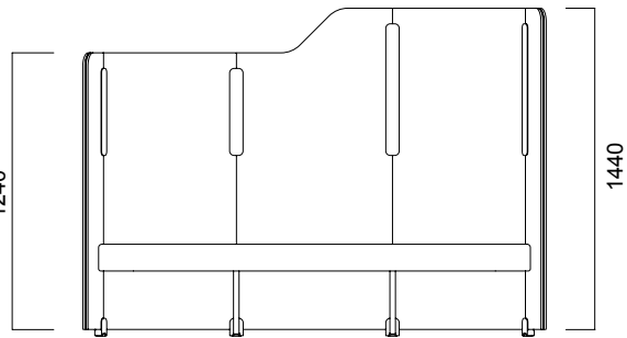
Tip 1 Açılı Tekli Kademeli Panel
